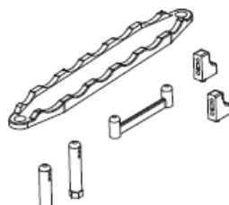
Cales + fixation batterie - S10
