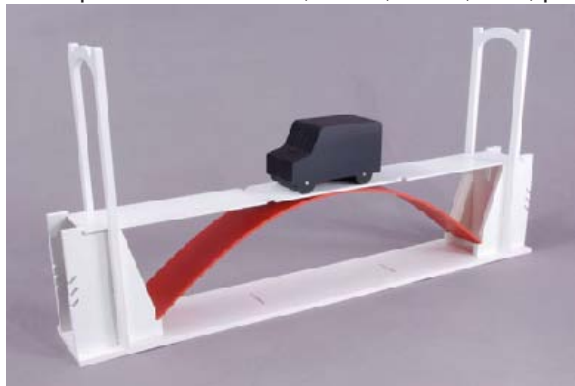
5 - Maintien par une voûte
