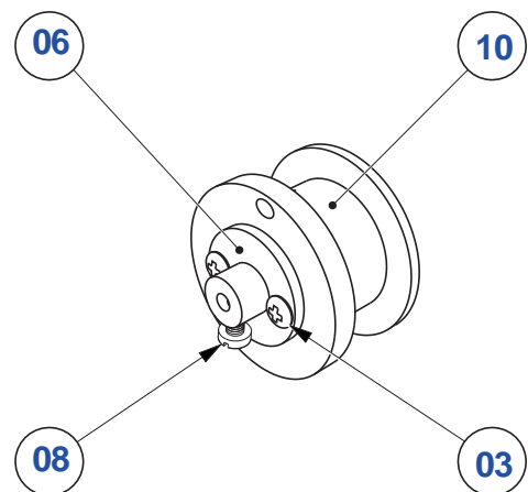
Poulie
