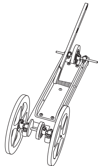
Banc d'essais avec poulie Ø 3 mm
